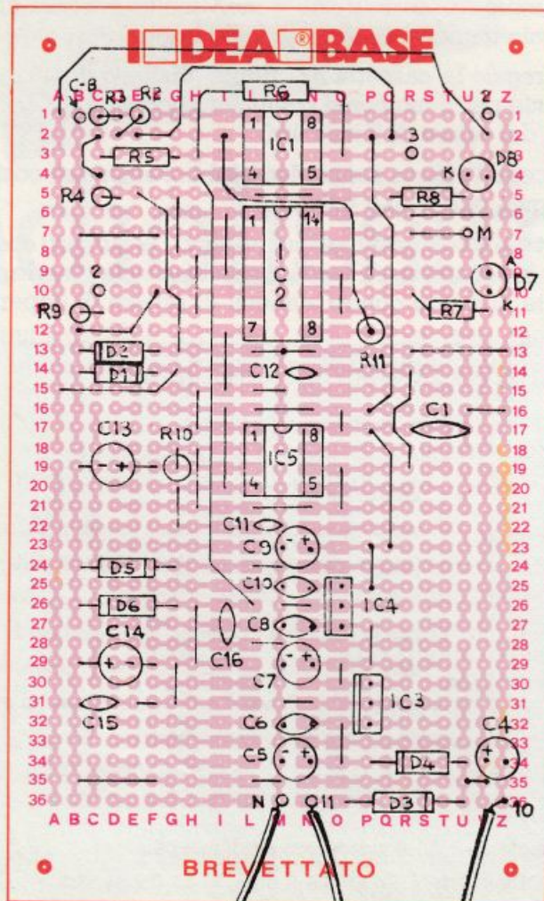
Figura 3. Lo schema di cablaggio dei componenti.
